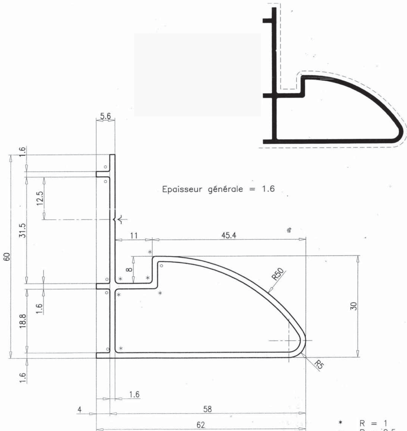
Profil Mural Inférieur (Blanc 9010)
